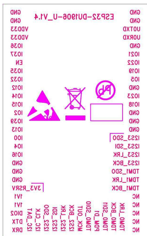
ESP32-DU1906-U
