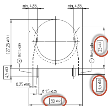
actual drawing 3.8755.4-1
