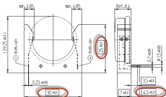
actual drawing 3.8756.4-1
